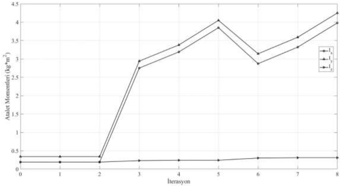
Şekil 6: Atalet momentleri
