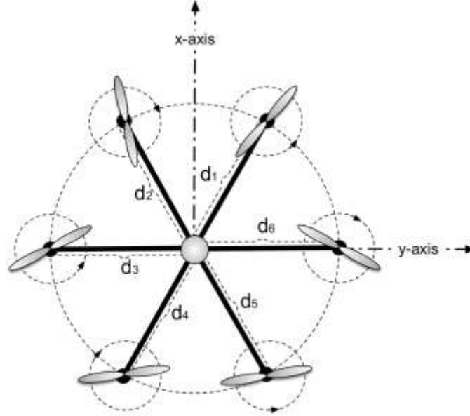
Şekil 1: Hexarotor model 1
