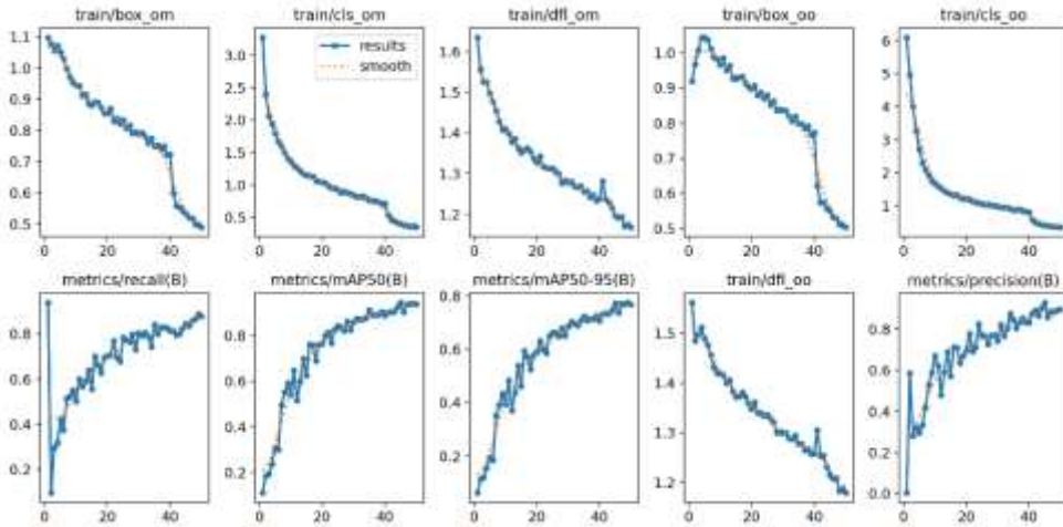
Şekil 4. YOLOv10 ağı ile eğitilen modelin başarı metriklerine ait grafikler.
