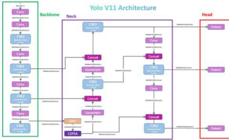
Şekil 2. YOLOv11 ağ mimarisi (Rao, 2024).
