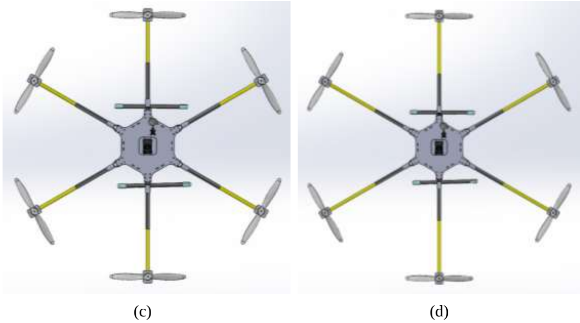
Şekil 2: Hexarotor başkalaşım (a) 37 cm kol uzunluğu, (b) 45 cm kol uzunluğu, (c) 55 cm kol uzunluğu ve (d) 65 cm kol uzunluğu.
