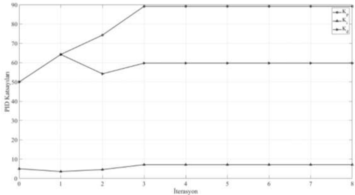
Şekil 7: PID katsayıları
