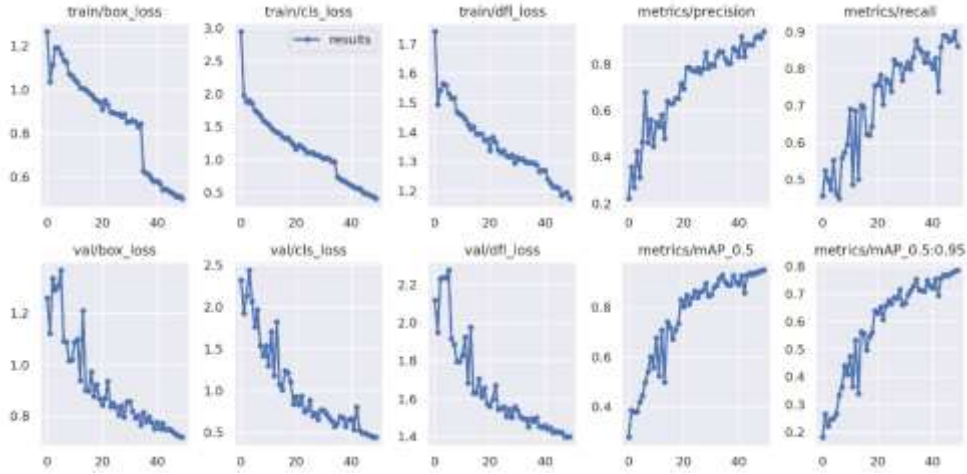
Şekil 3. YOLOv9 ağı ile eğitilen modelin başarı metriklerine ait grafikler.
