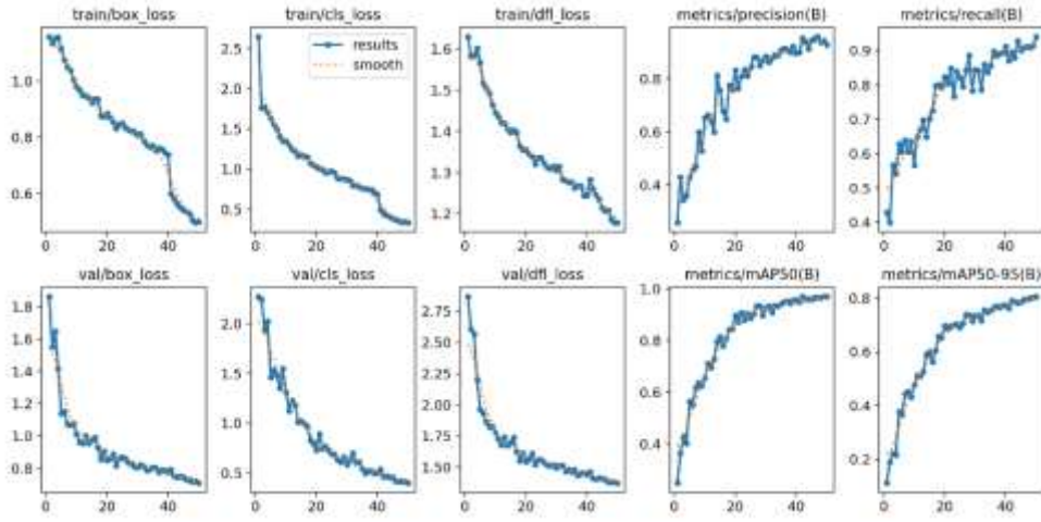
Şekil 5. YOLOv11 ağı ile eğitilen modelin başarı metriklerine ait grafikler.
