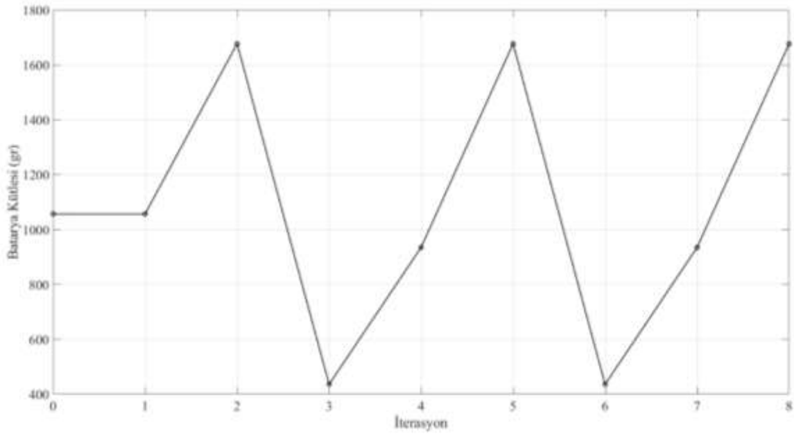
Şekil 4: Batarya kütlesi
