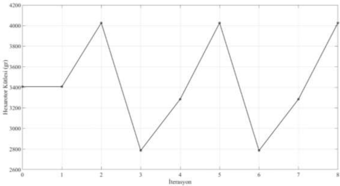
Şekil 5: Hexarotor kütlesi
